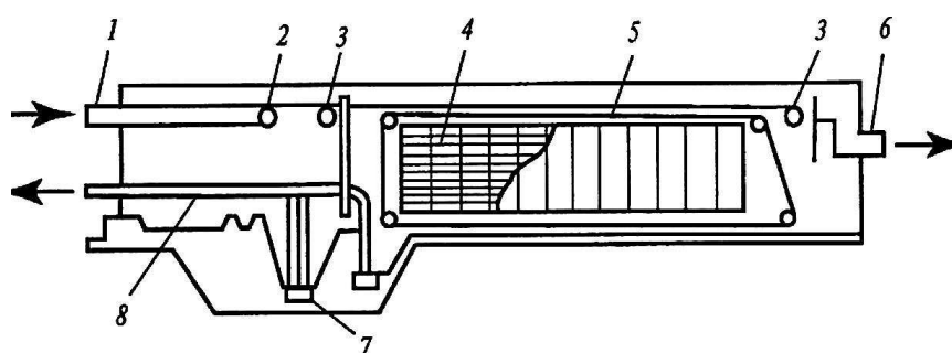
Рисунок 4.2 – Горизонтальная жируловушка:
