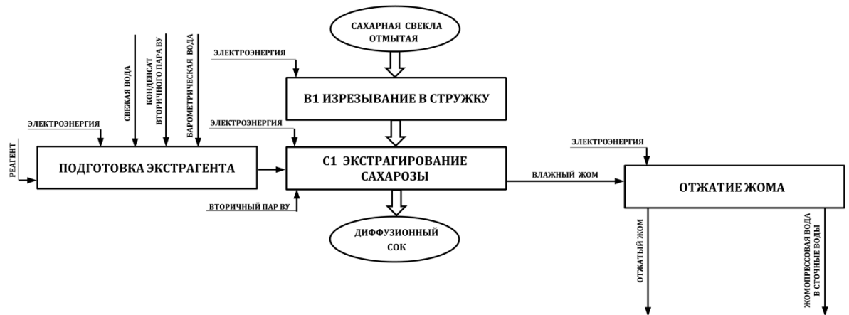
Рисунок 2.28 – Структурная блок-схема процесса получения диффузионного сока
